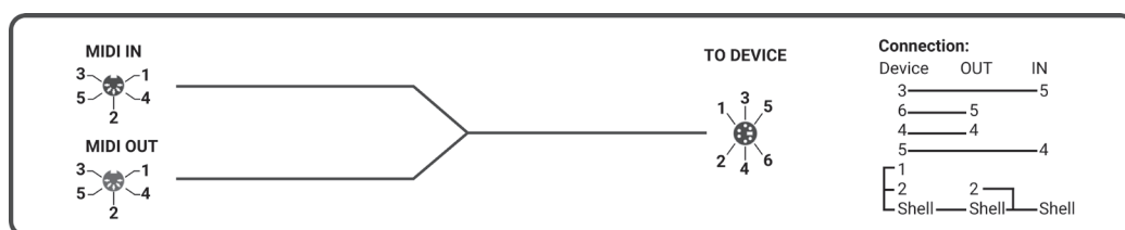
図 1. MIDI ブレイクアウト・ケーブル配線図
